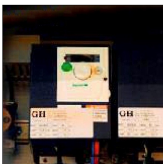
12 Frequenzumrichter Längsfahrt
